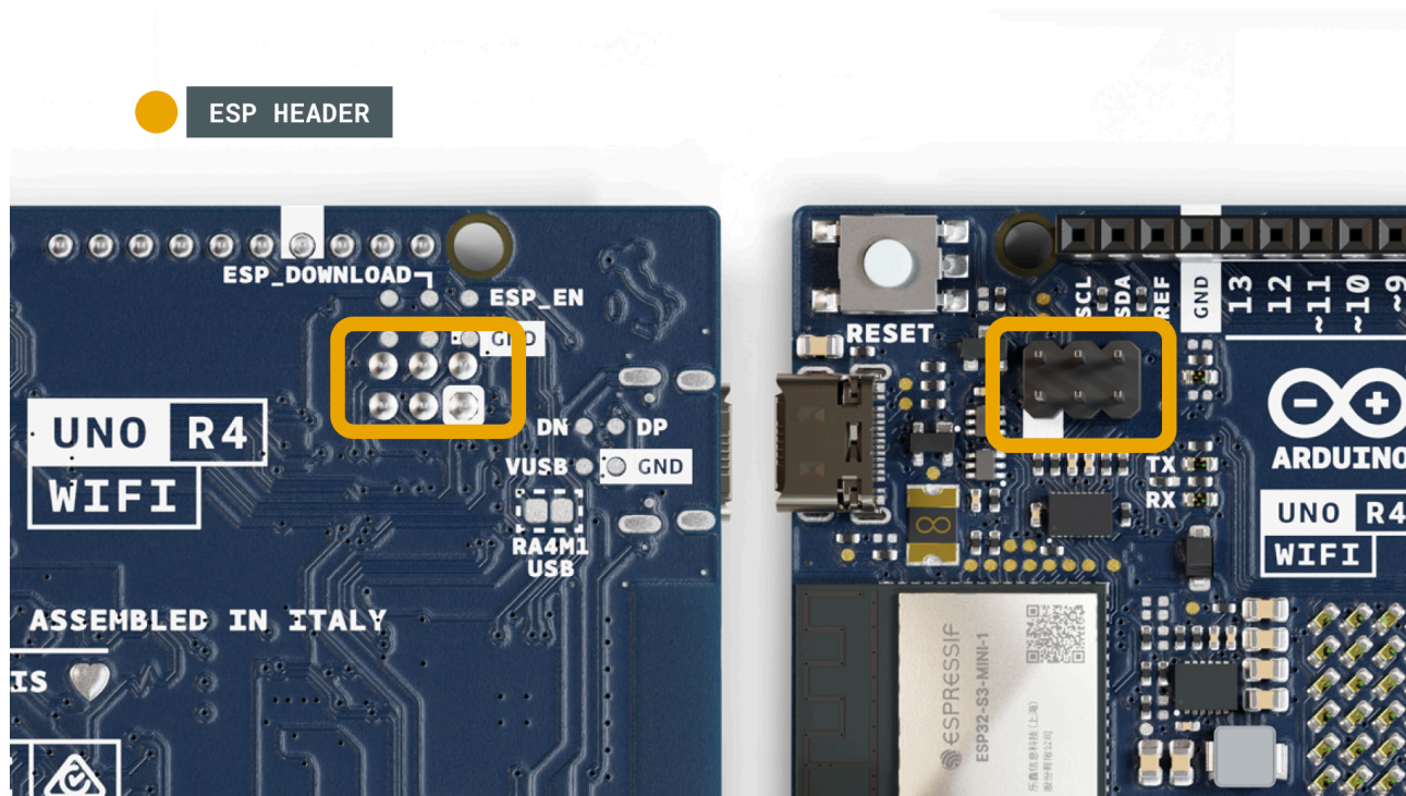
ESP针脚
